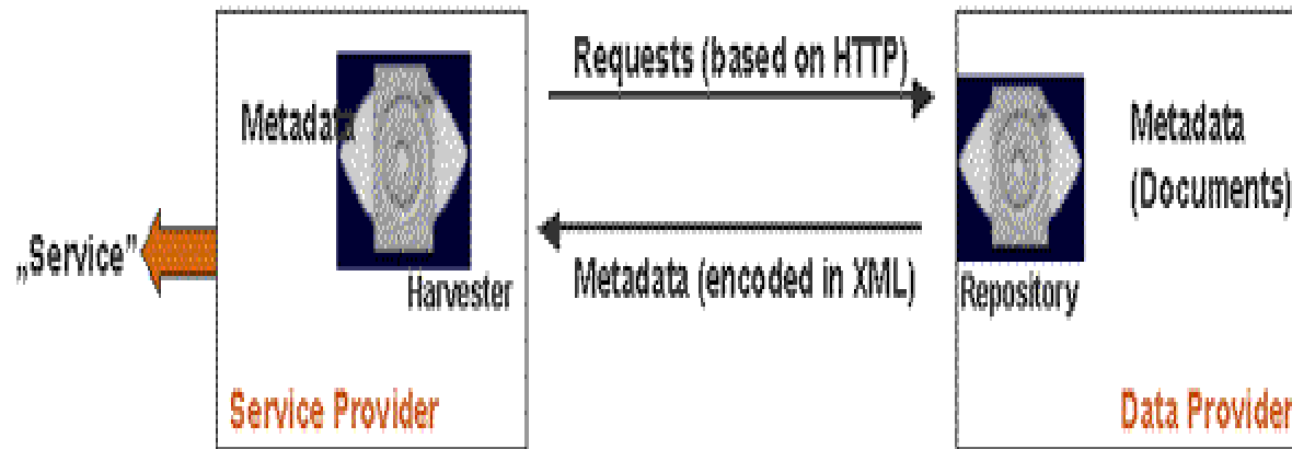
Figura 1 Estructura básica del modelo OAI-PMH
