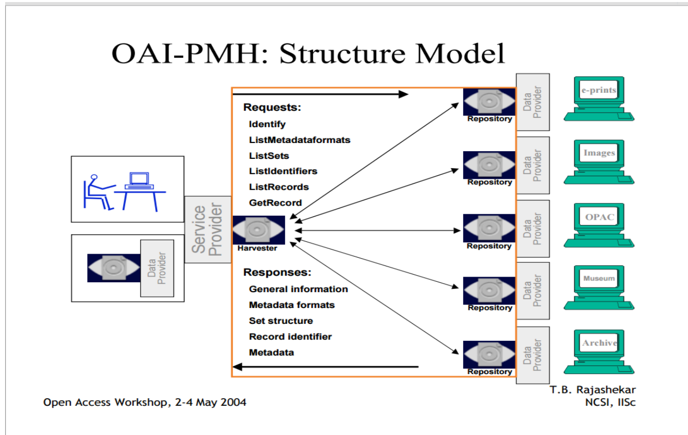
Figura 6 Modelo Estructural OAI-PMH
